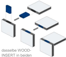
Abb. 1 mit Holzdübel verleimte Korpusecke
