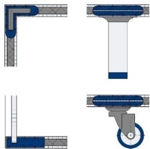
Abb. 3 Gehrungsecke, Rückwandanschluss und Schraubmontage von Anbauteilen
