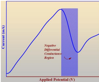
Arbeitsbereich der Resonanztunnel diode
