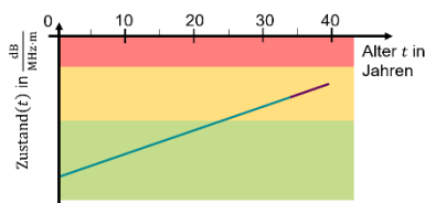
Zustandsgerade zur Bewertung der Kabelqualität
