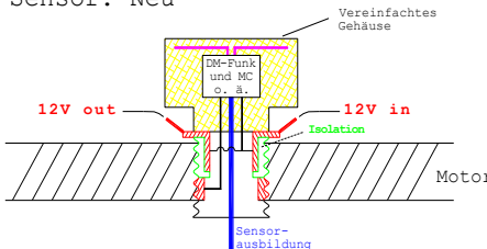
Aufbau eines Funksensors im Motor
