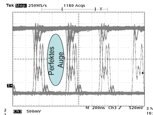
Messdaten eines 2,45 GHz-Prototypen mit einer Übertragungsstrecke im Motorraum
