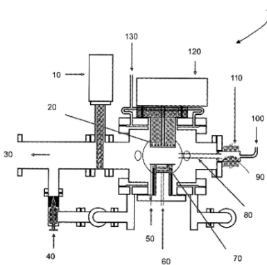
Beispielhafte Darstellung einer geeigneten Gasphasenabscheidungsanlage
